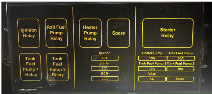
Fuse Box – LT4
